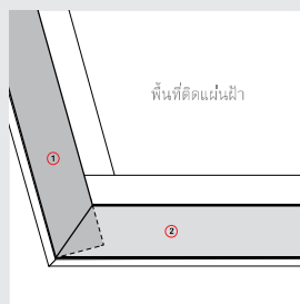
การติดตั้งคิ้วฝ้าเข้ามุมนอก กรณีทำมุมมากกว่า 90°
